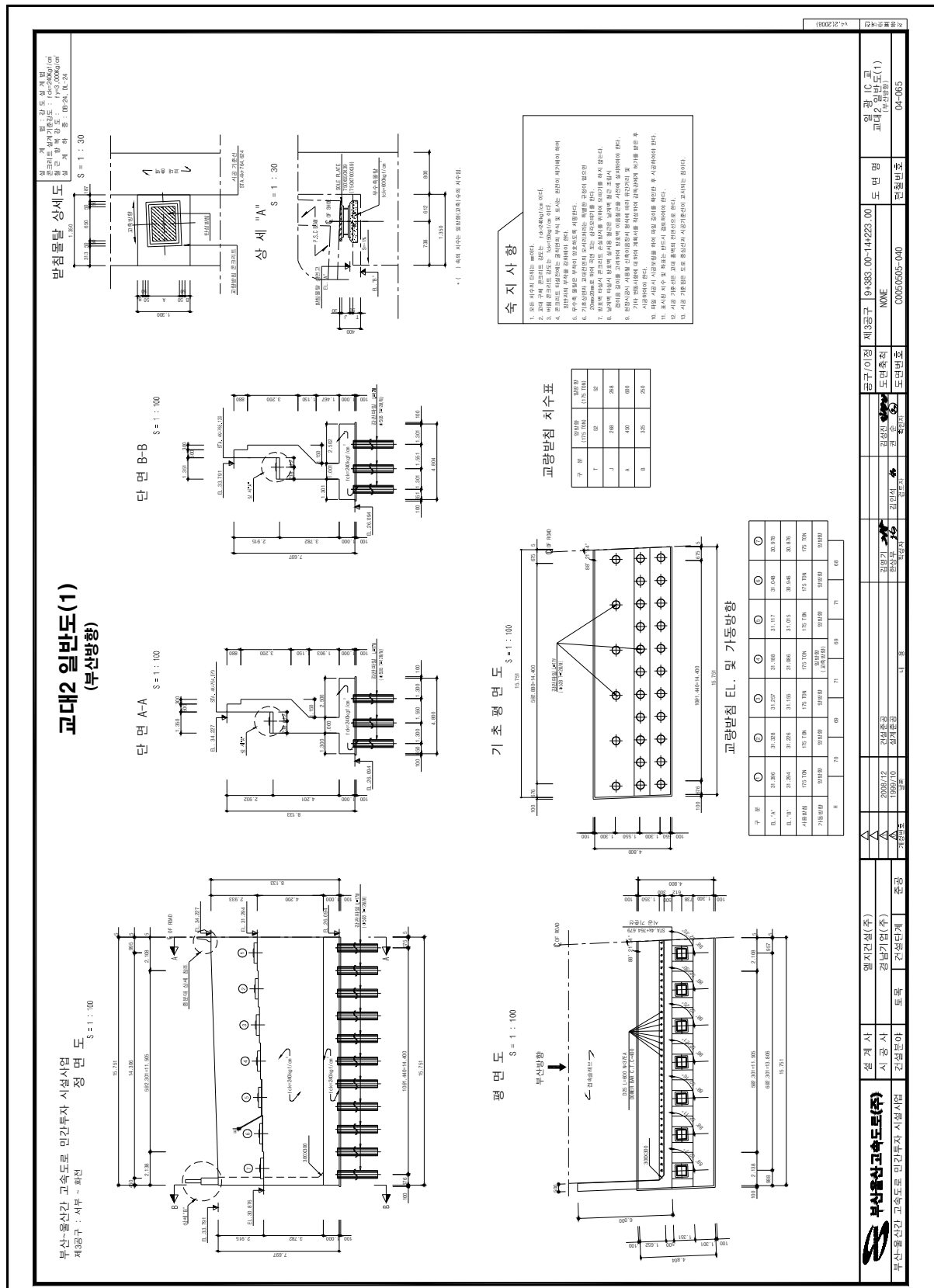
【그림 38.1.5】 교대 일반도(계속)
