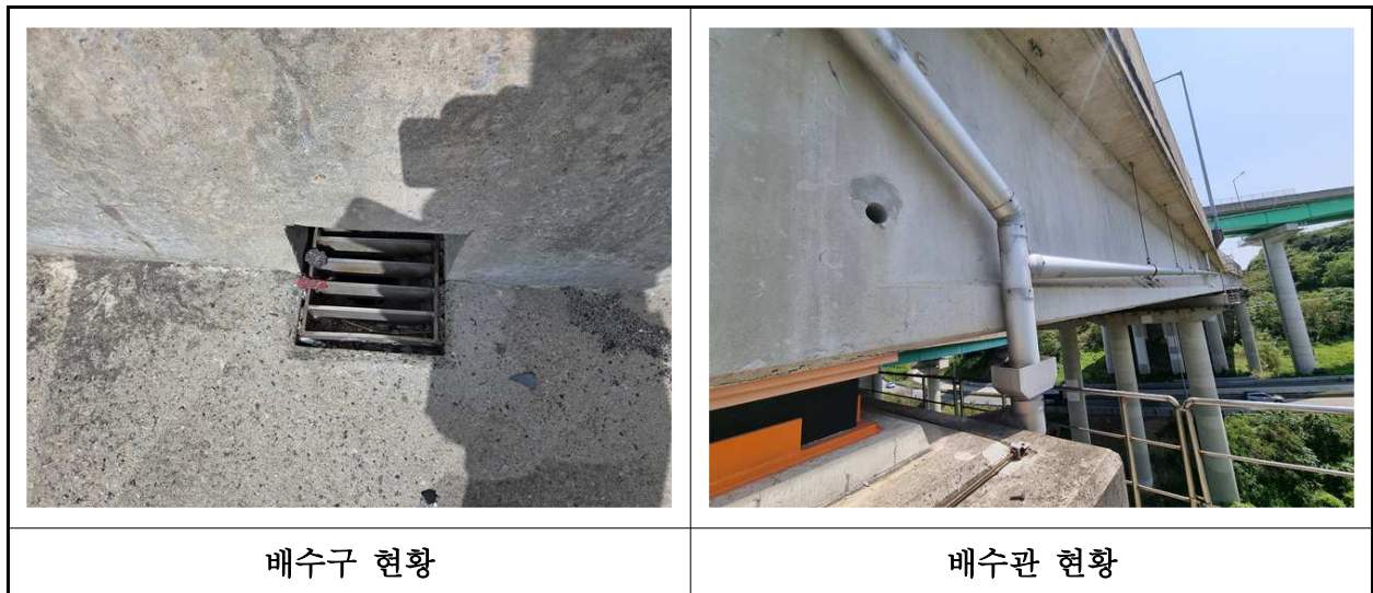
【사진 38.3.22】 배수시설 전경
