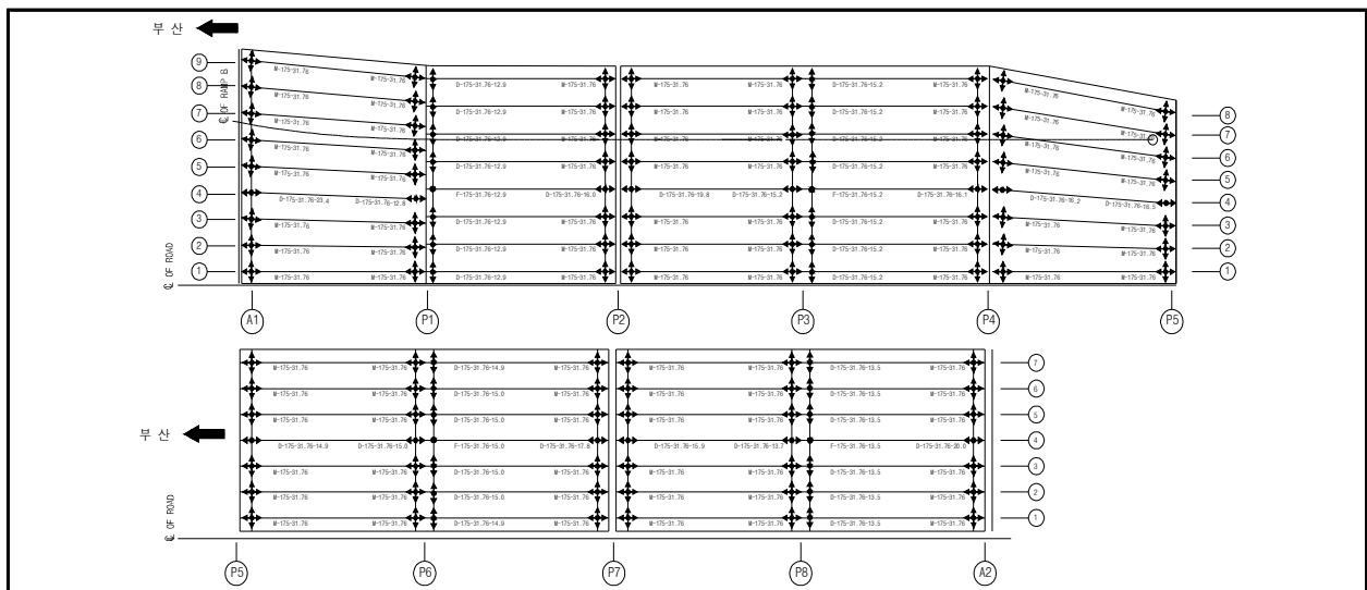
【그림 38.3.1】 교량받침 배치도
