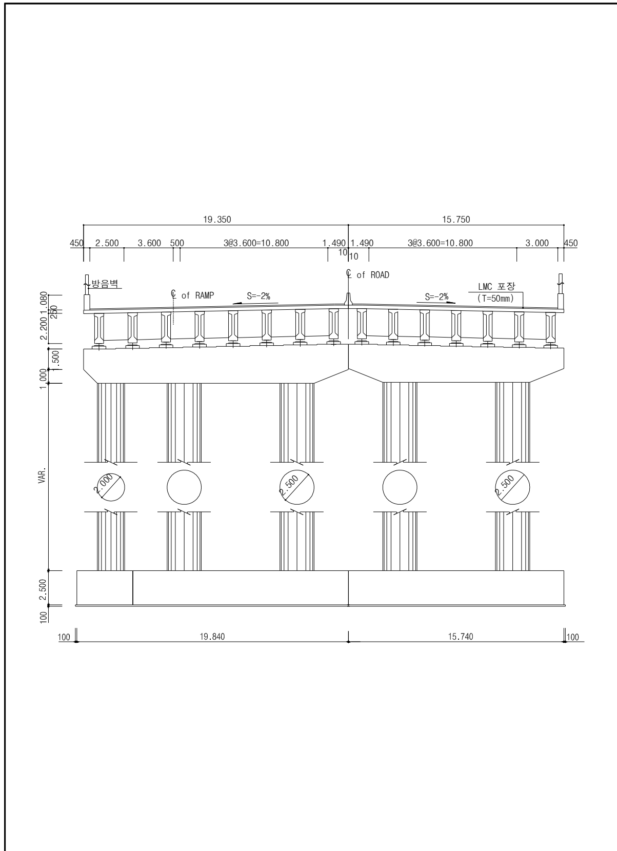
【그림 38.1.3】 횡단면도
