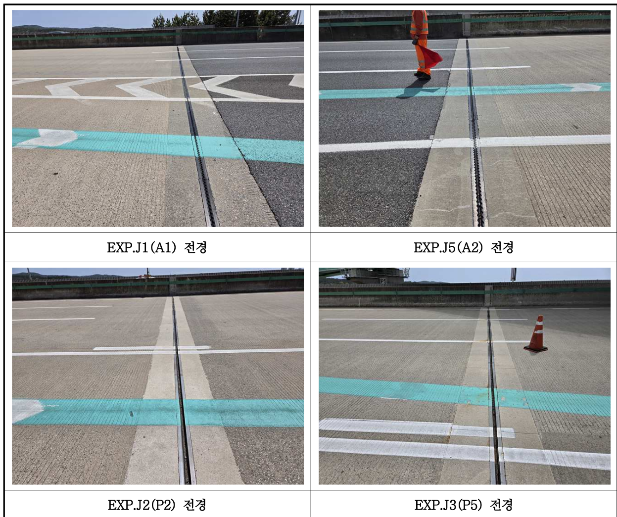
【사진 38.3.17】 신축이음장치 전경
